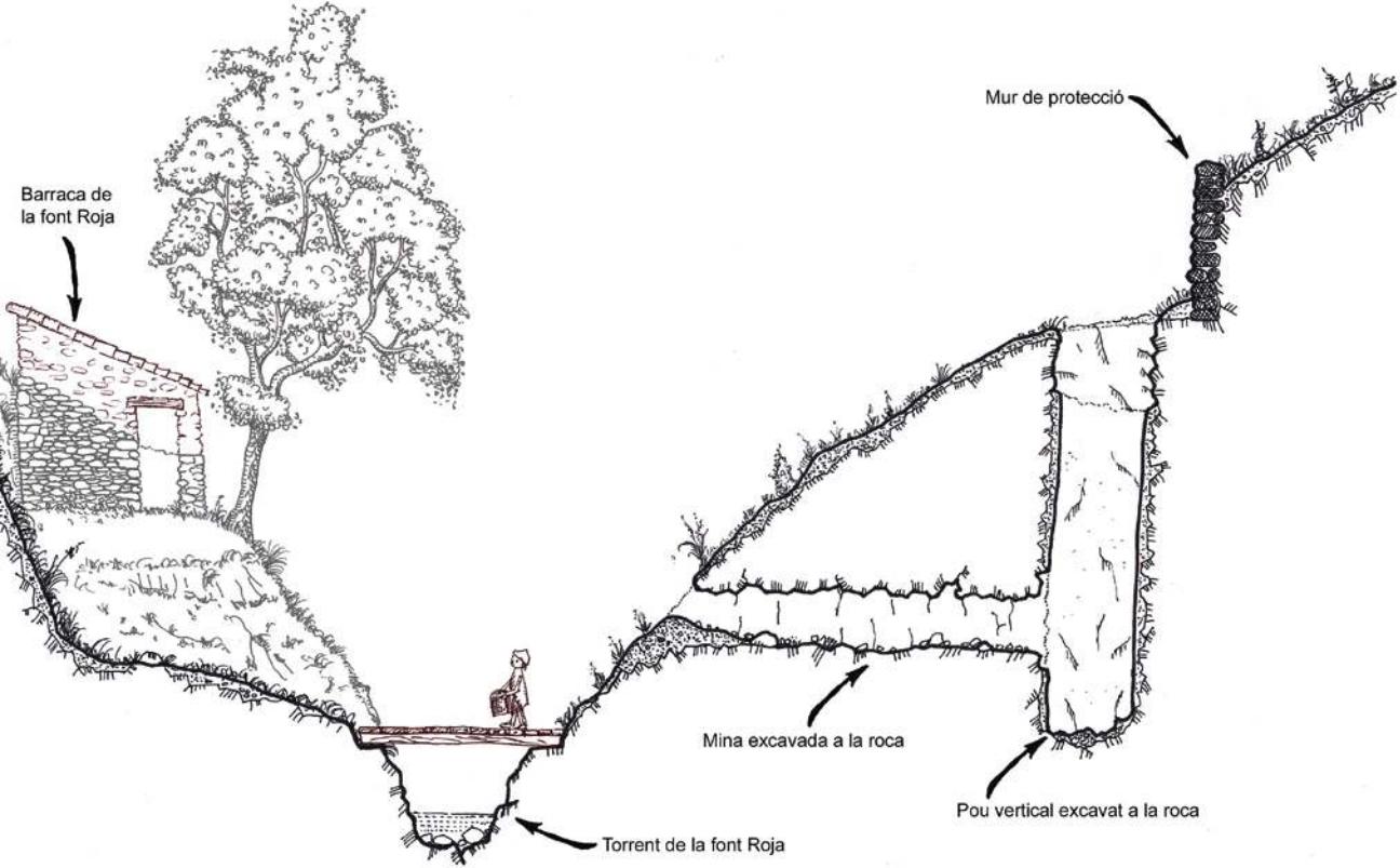
Esquema del pou de cata de la font Roja
